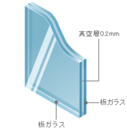
真空ガラス構造図
